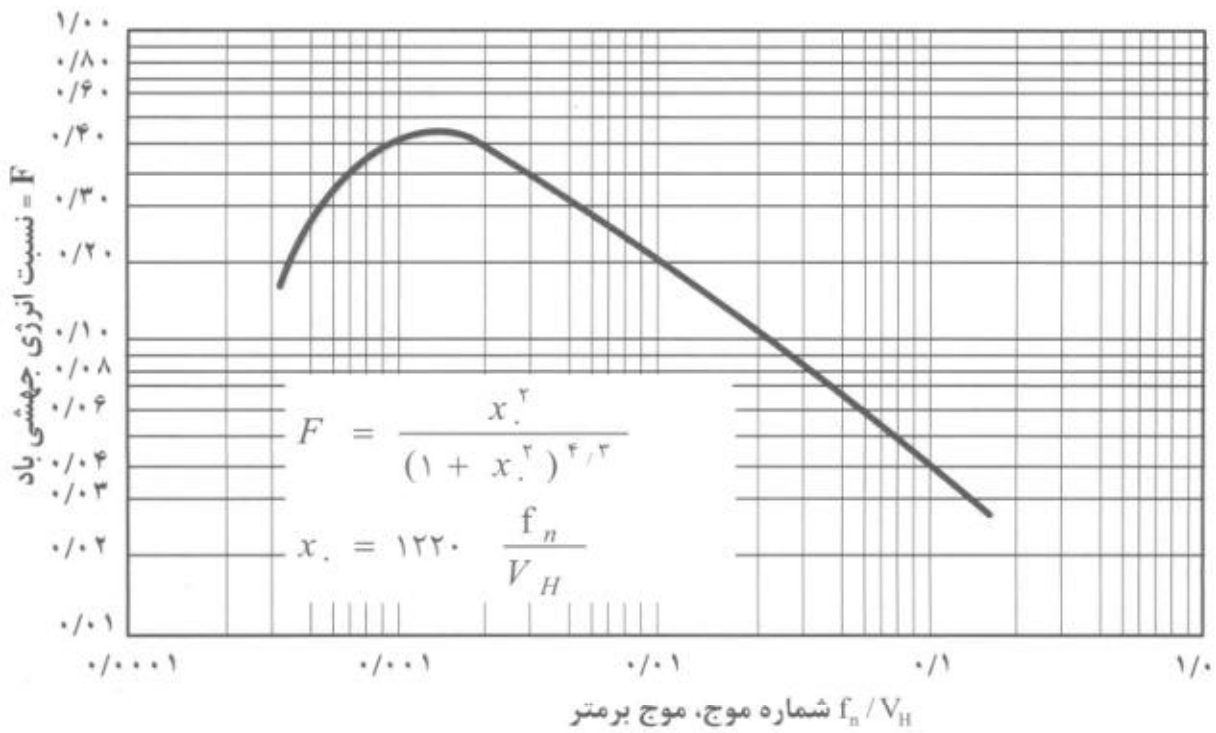
شکل پ-۲-۶-۴ نسبت انرژی جزئی باد بعنوان تابع تعداد موج
